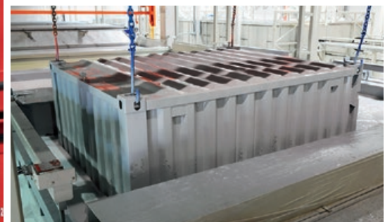
KTL-Grundierung im Tauchbecken
